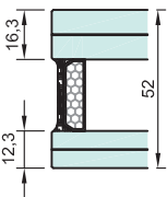
CRISTAL CÁMARA ACÚSTICO altas prestaciones hasta R_w (C; Ctr): 51(-1, -4) \text{ dB} ISO 717-1
