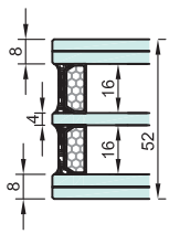
CRISTAL DOBLE CÁMARA, máximo aislamiento térmico U_w = 0.5 \text{ W}/(\text{m}^2 \text{ K})
