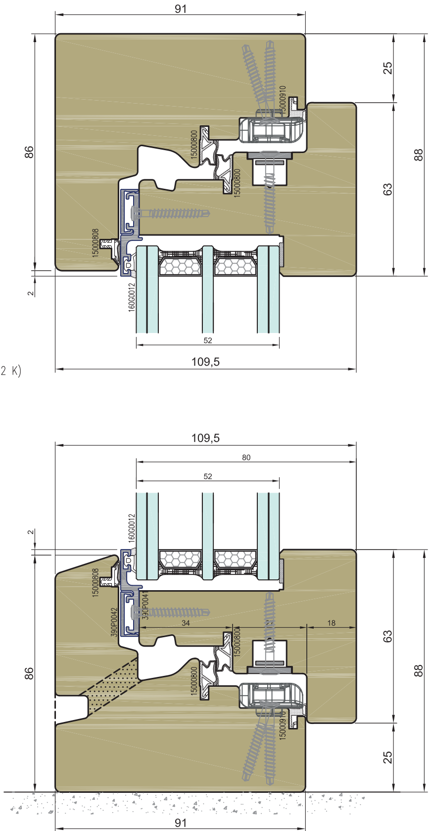
CRISTAL CÁMARA ACÚSTICO altas prestaciones hasta R_w (C; Ctr): 51(-1, -4) \text{ dB} ISO 717-1
